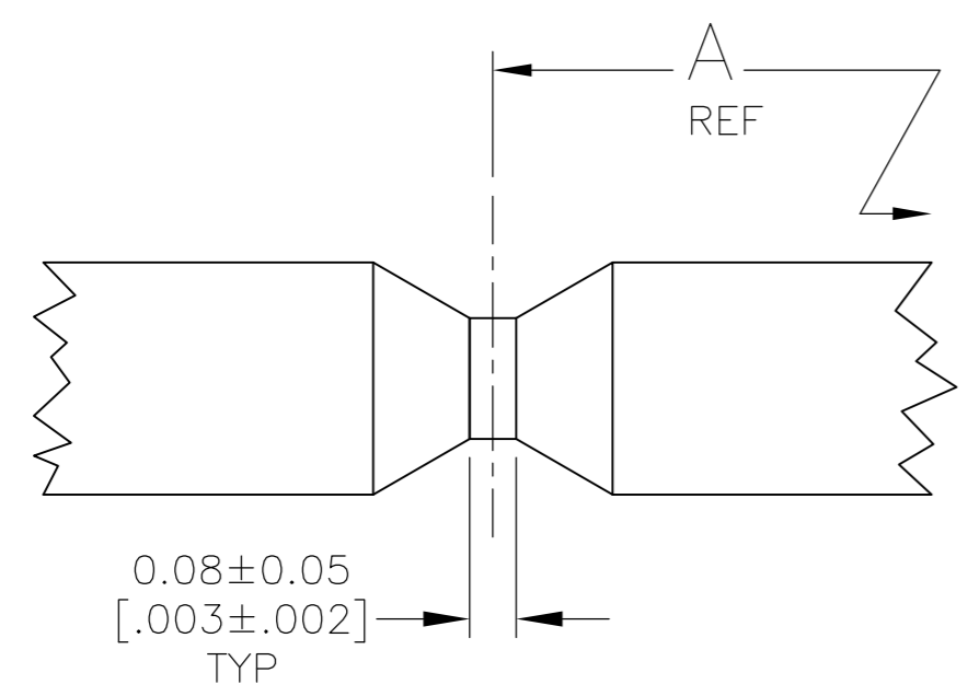
DETAIL W 30:1
